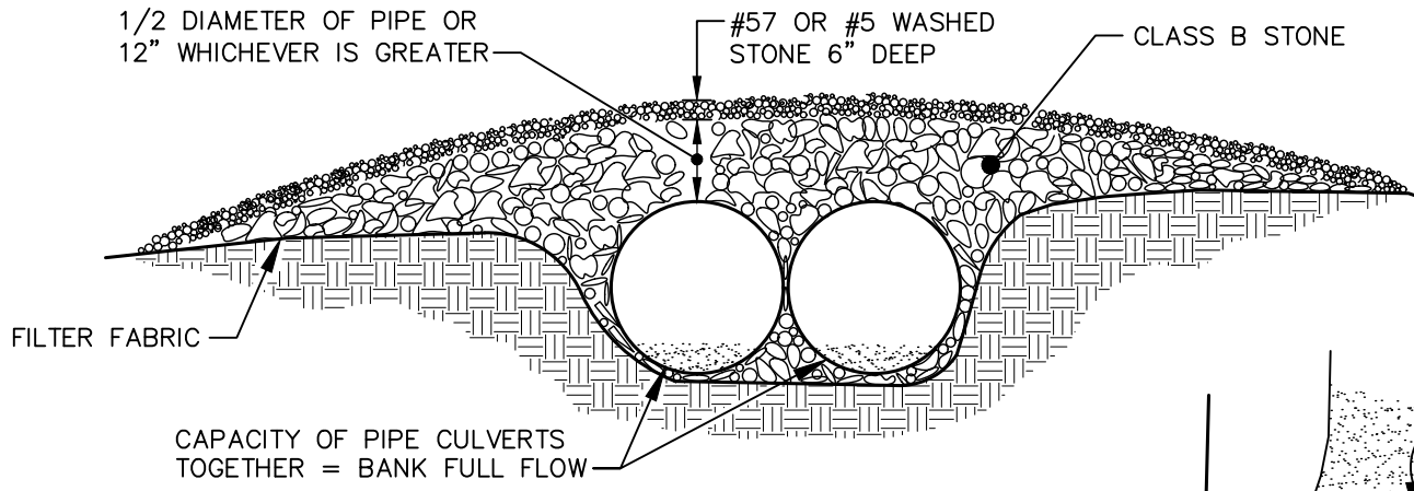
ELEVATION
