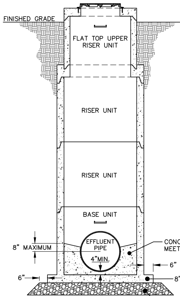
SECTION A-A
