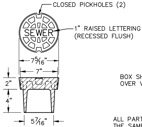
LID
