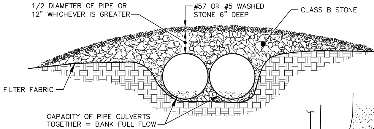
ELEVATION
