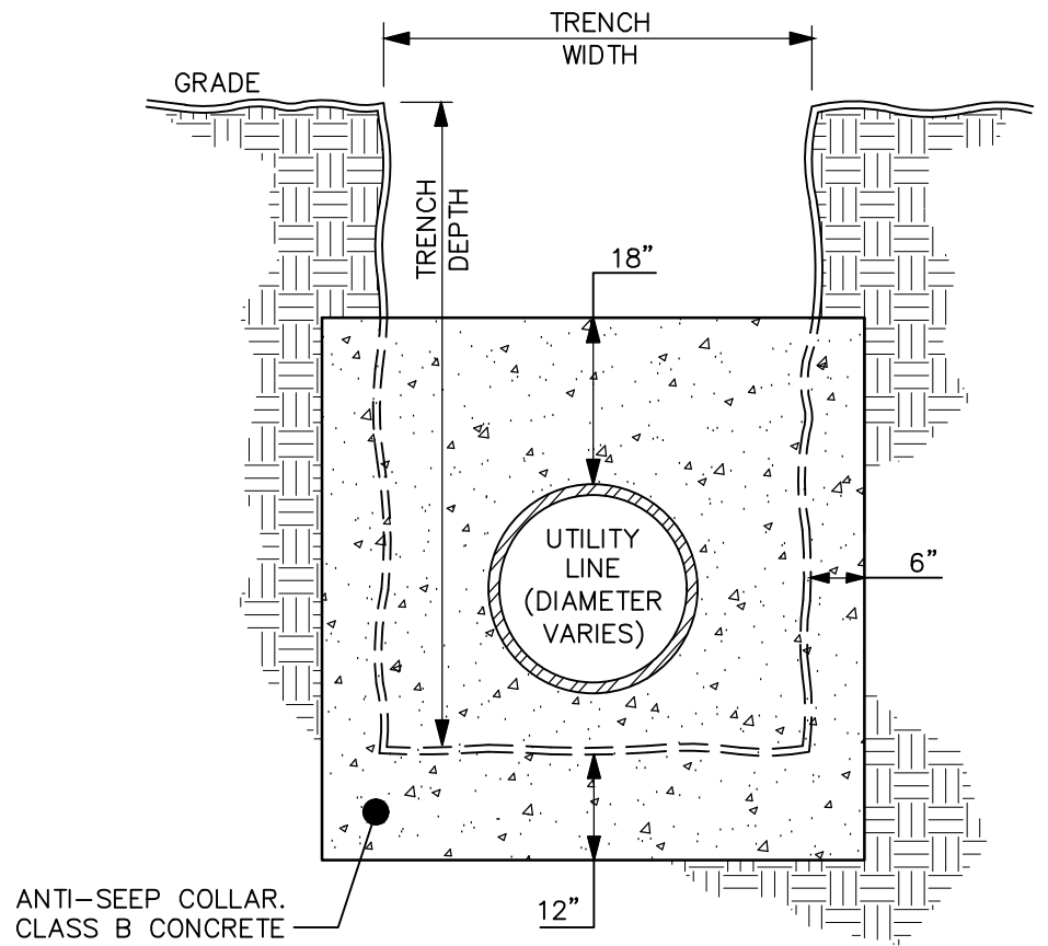
SECTION A-A
