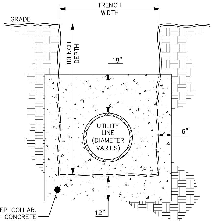
SECTION A-A
