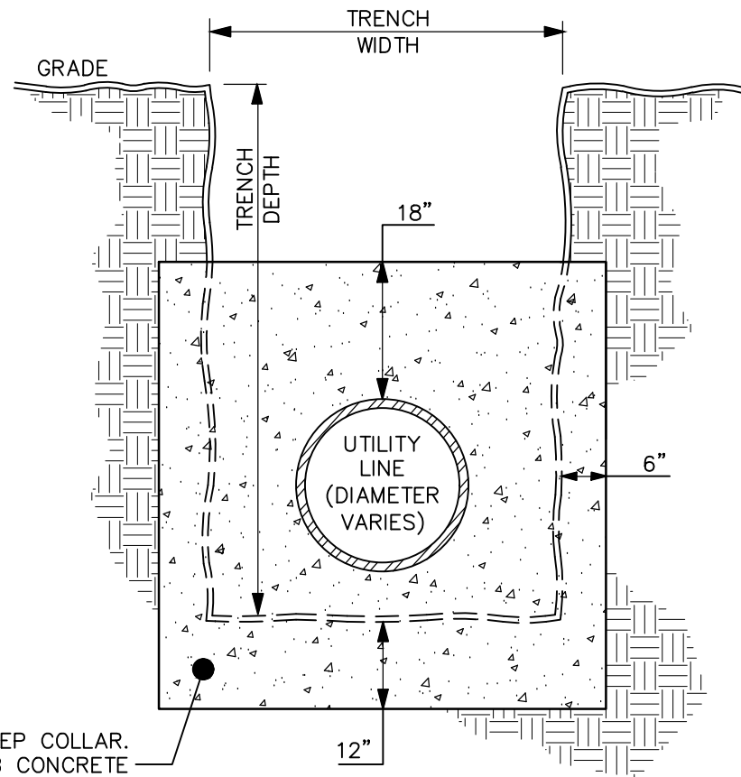
SECTION A-A
